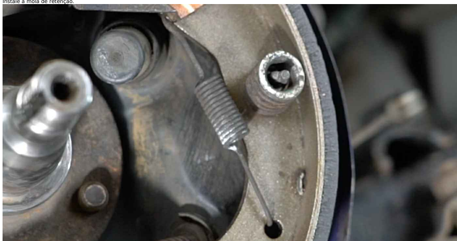
40 Instale a mola de retorno superior. Utilize um alicate de ponta longa.
